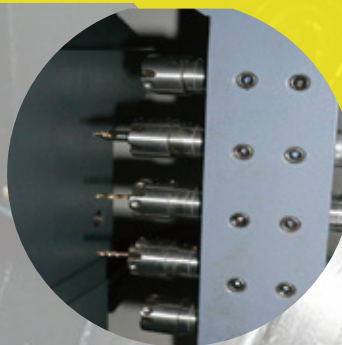
端面三軸動力裝置 (ER-20) End side live tooling device(4-shaft)
