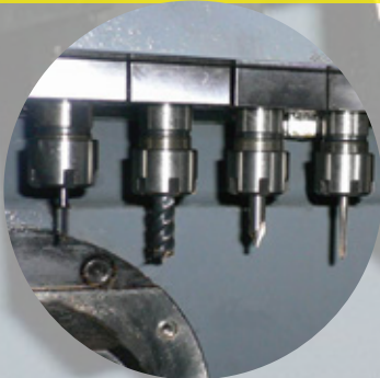
側銑四軸動力裝置 (ER-16) Cross side live tooling device
