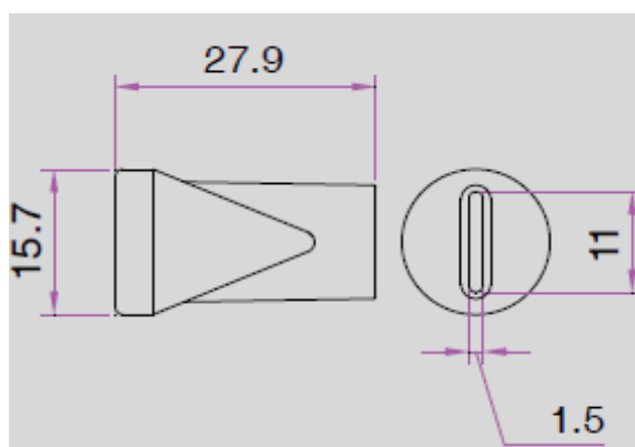
Чертеж сопла плоского 82075
