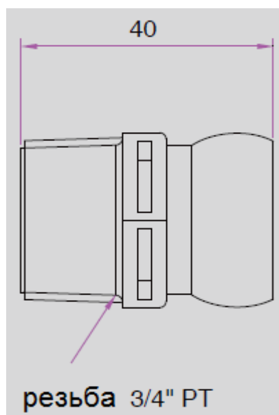
Чертеж соединителя 86074
