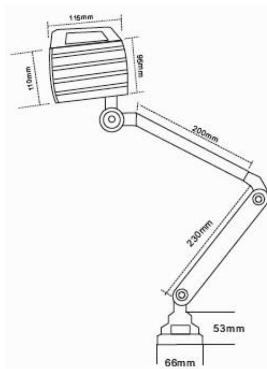
Чертеж светильника FL12-24L
