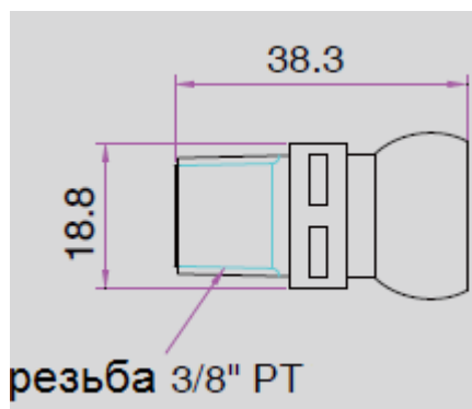
Чертеж соединителя 84066
