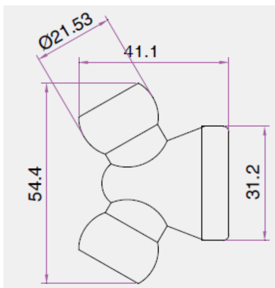
Чертеж переходника Y-образного 86079
