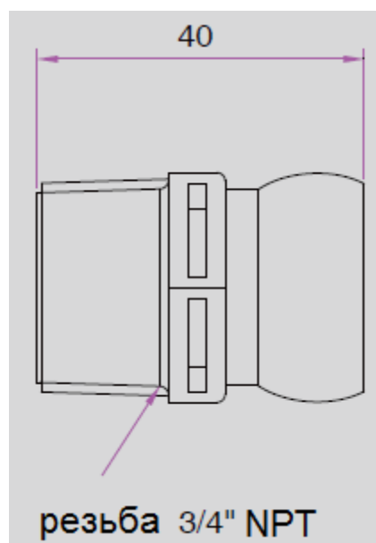
Чертеж соединителя 86074А
