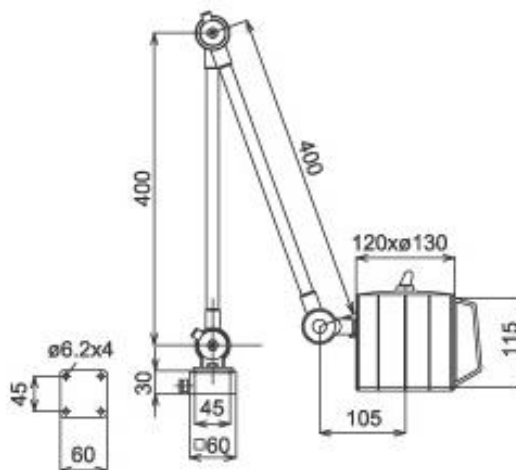
Чертеж светильника G-L75
