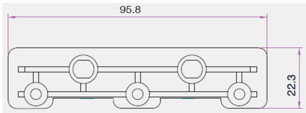
Чертеж основания распределителя 54416
