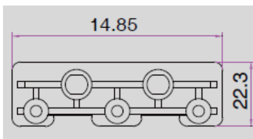
Чертеж основания распределителя 52416
