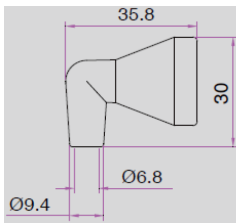
Чертеж сопла углового 84463
