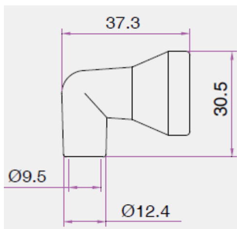
Чертеж сопла углового 84464
