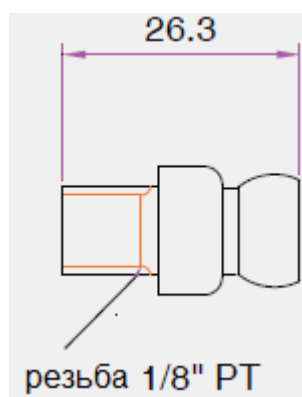
Чертеж соединителя 82035
