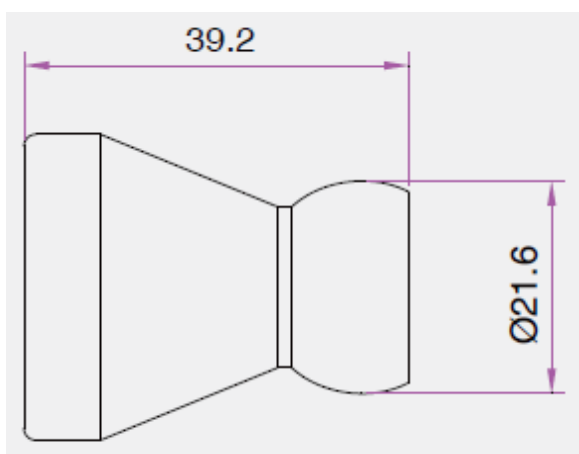
Чертеж переходника 86071
