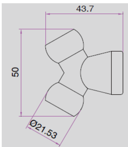
Чертеж соединителя Y-образного 84068
