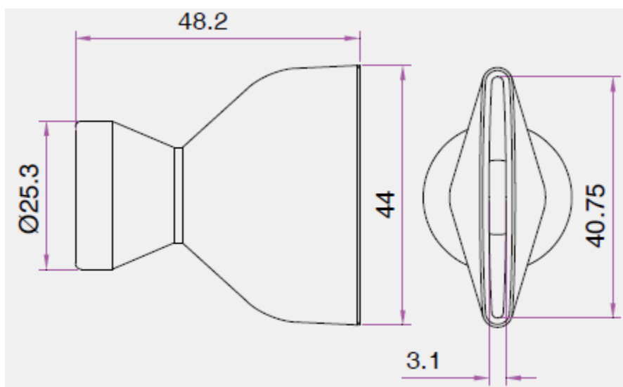
Чертеж сопла плоского 84079
