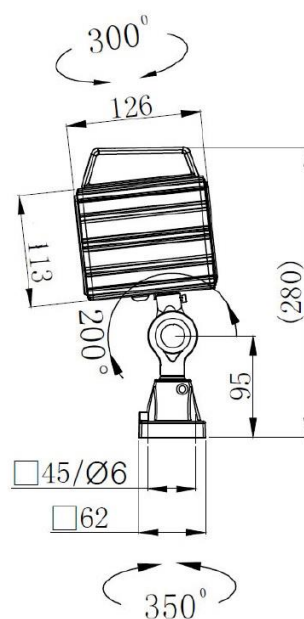
Чертеж светильника ST-L24-S95
