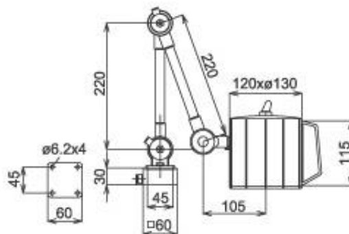
Чертеж светильника G-M75
