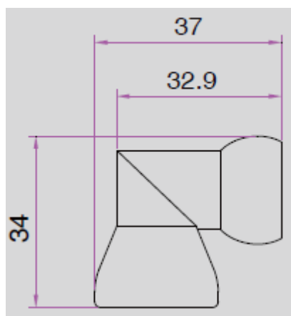
Чертеж соединителя углового 64640
