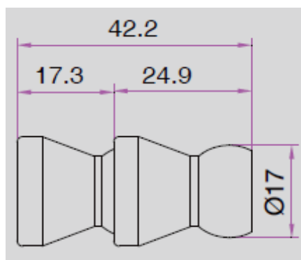
Чертеж двух звеньев 83091 в сборе
