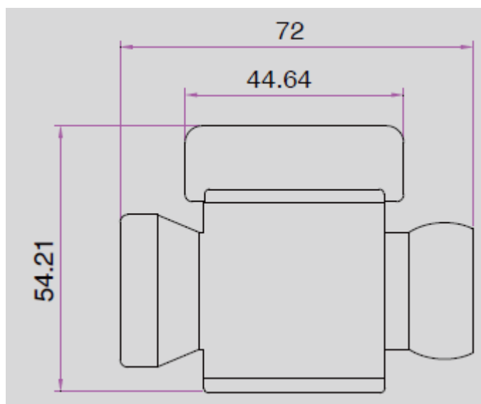
Чертеж крана проходного 86742
