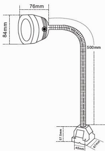
Чертеж светильника
