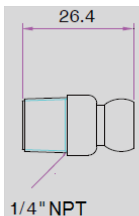
Чертеж соединителя 82036А
