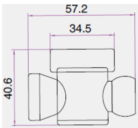
Чертеж крана проходного 84742
