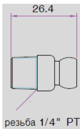
Чертеж соединителя 82036
