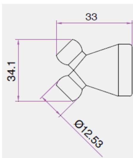
Чертеж переходника Y-образного 84069
