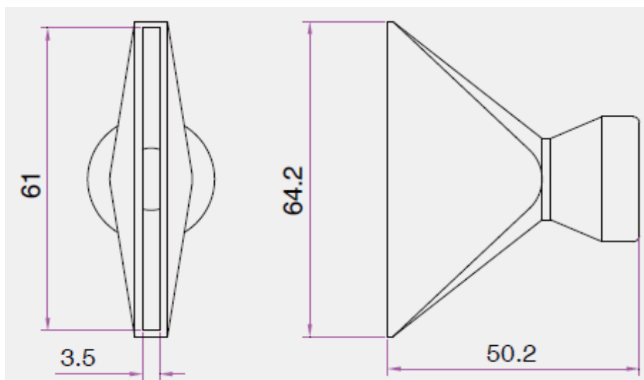
Чертеж сопла плоского 84072
