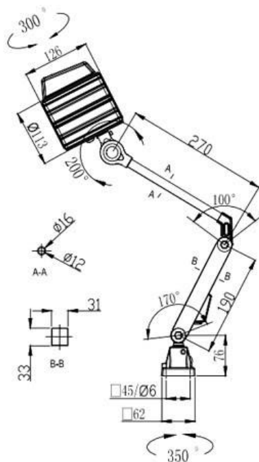
Чертеж светильника ST-L24-M95
