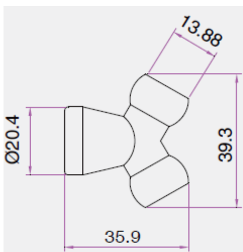
Чертеж соединителя Y-образного 83058
