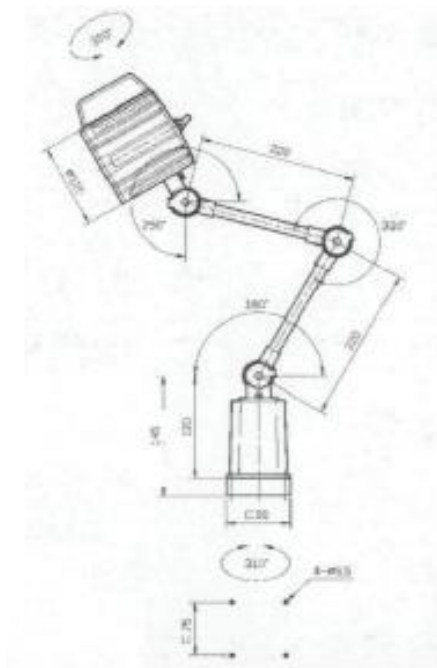
Чертеж светильника JW-55RTL
