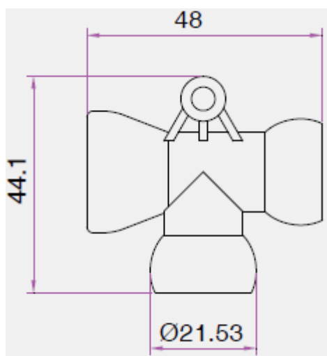
Чертеж соединителя Т-образного 64646
