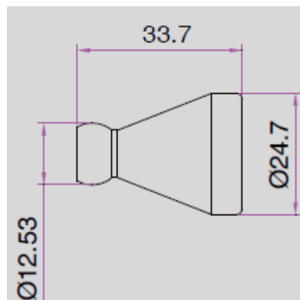
Чертеж переходника 84851
