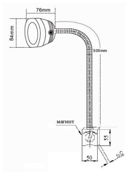
Чертеж светильника
